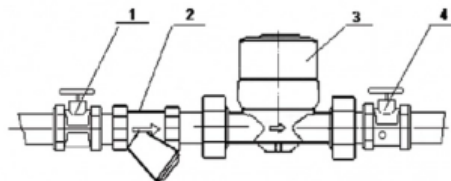
Схема водомерного узла. 1. Кран шаровой. 2. Фильтр. 3. Счетчик. 4. Кран шаровой со сливом.
